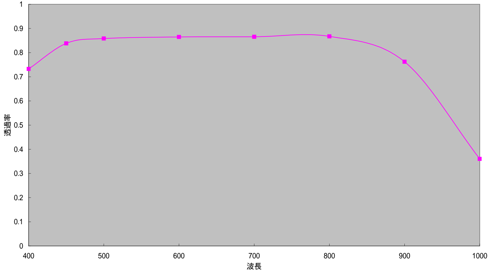
LM16JC10M 透過率
