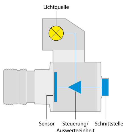
Abbildung 1 - Komponenten der Time-of-Flight-Kamera.
