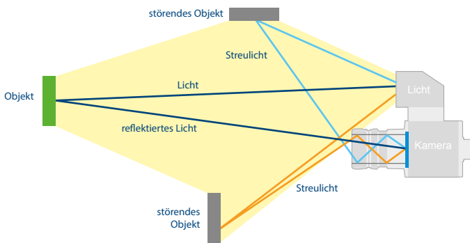
Abbildung 5 - Streulicht
