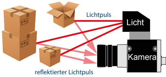
Abbildung 2 - Funktionsprinzip der Lichtlaufzeit-Kamera.
