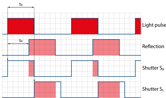
Abbildung 3 - Belichtungszeit
