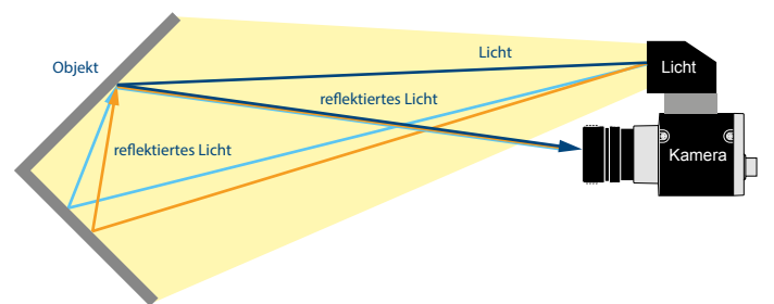
Abbildung 4 - Mehrfach-Reflexion
